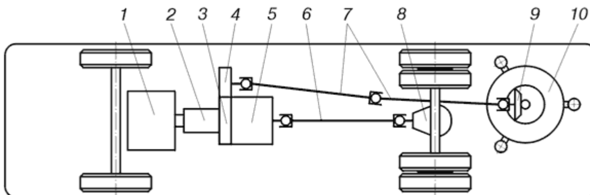
Рис. 3. Схема городского электробуса новой концепции:
