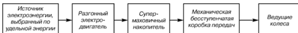
Рис. 2. Схема электрооборудования нового концепта
